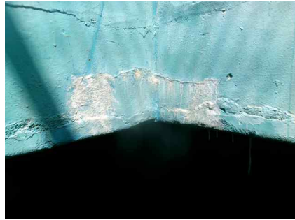
<배수지 1지 상부슬래브 백태>
